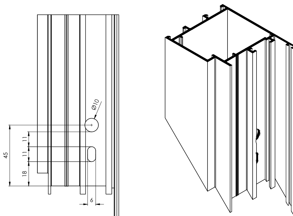
Mecanizado Hoja 3041 para escuadra E70 + E67
