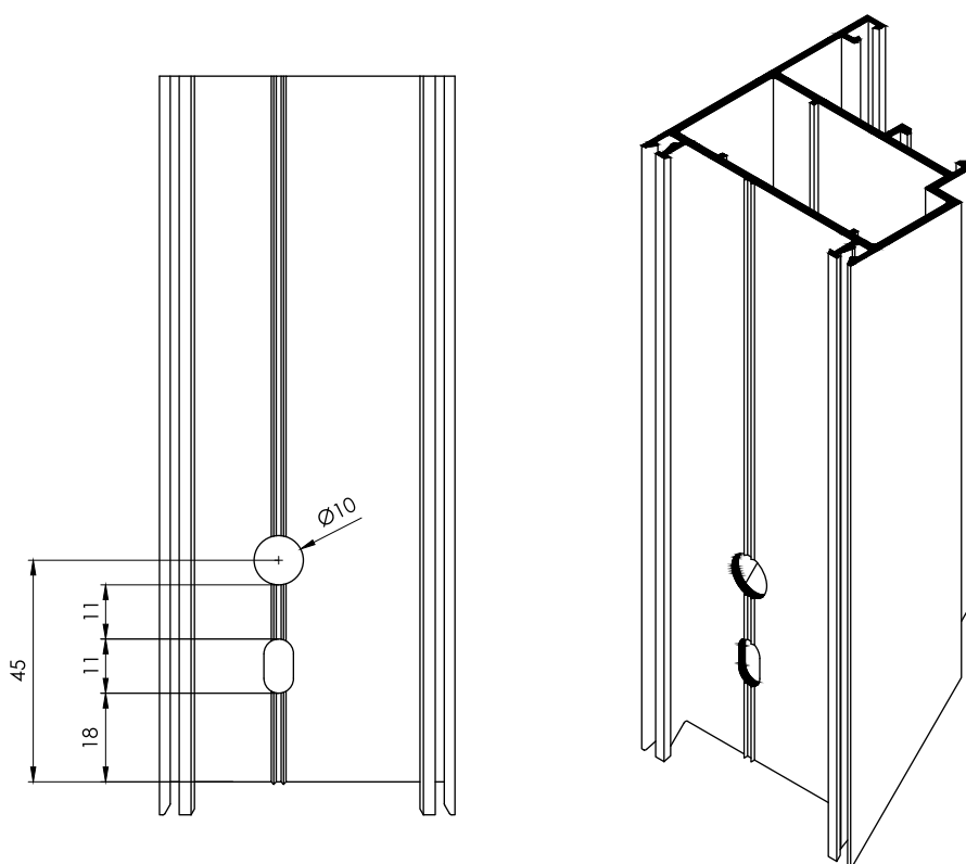
Mecanizado Marco 3040 para escuadra E70
